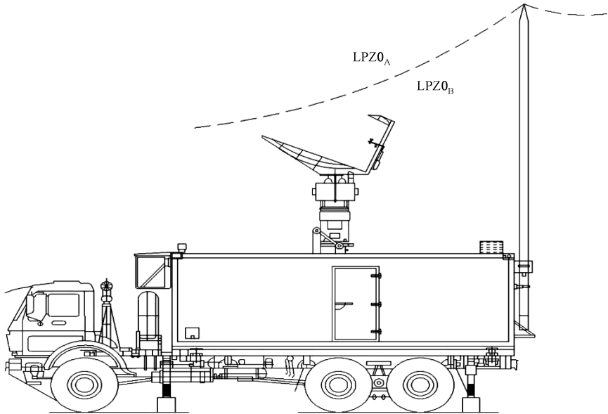
图 C.1 移动设施接闪杆保护范围示意图
