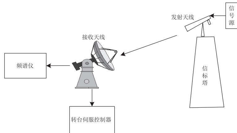
图 13 天线交叉极化隔离度测试示意图
