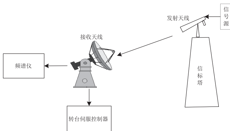
图 10 天线第一副瓣电平测试示意图
